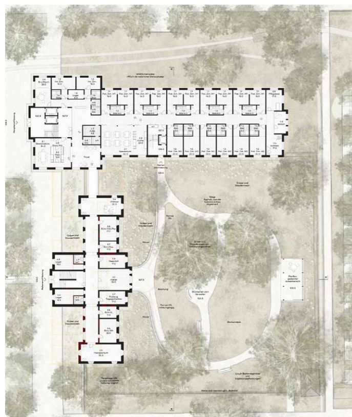
Grundriss EG
