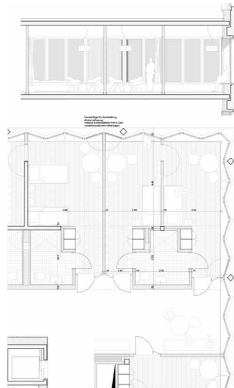
Grundriss Ausschnitt 1:50
